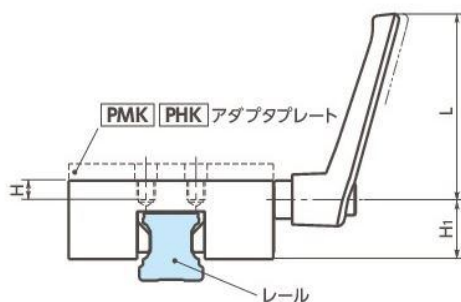
図 1. 寸法表記載の寸法図
