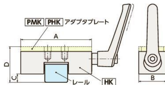
図 2. 選定表記載の寸法図
