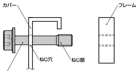
SSC-SFSS フランジ付き六角穴付き脱落防止ねじ
