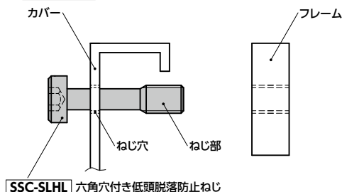
SSC-SLHL 六角穴付き低頭脱落防止ねじ
