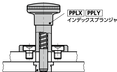
PJB 位置決めピン用ブッシュ
