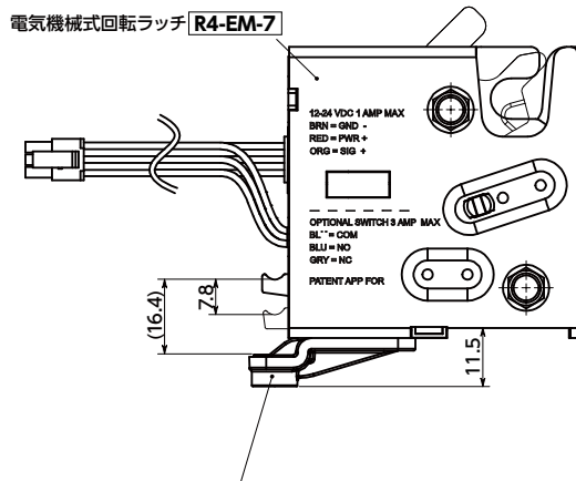
電気機械式回転ラッチ用ワイヤ取り付けキット R4-EM-52
