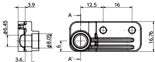
断面図 A-A'
