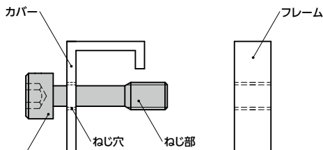
SSC-RY 六角穴付き脱落防止ねじ
