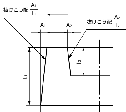
● 図 鑄鉄品及び鑄鋼品の抜けこう配
